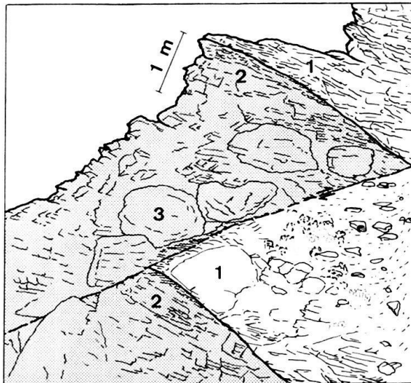
Fig. 7. Die Lagerungsverhältnisse des Dioritgangs vom Piz Val Gronda. 1 Nebengestein; verschieferte Zweiglimmer-Albit-Gneise. 2 Verschiefter, diaphthorierter Diorit. Stoffgrenze zum Nebengestein diskordant zur Schieferung, Schieferung des Diorits konkordant zur Schieferung des Nebengesteins. 3 Massiger, relativ gut erhaltener Diorit, in einzelnen Blöcken. Zusätzlich ist der Gang an einer Bruchfläche versetzt.
