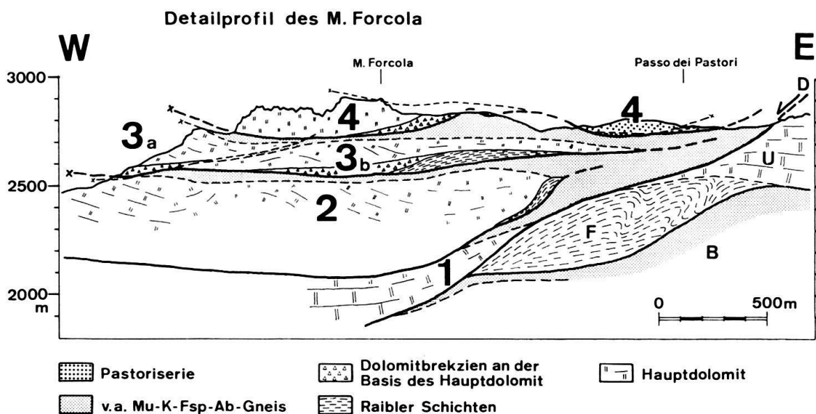
Fig. 19. Detailprofil des M. Forcola. 1 Rasch nach Norden und Osten auskeilender Quatervals-Hauptdolomit und Kristallin von Dössradond. 2 Unteres Stockwerk von Raibler Schichten, Hauptdolomit und Mu-K-Fsp-Ab-Gneisen. Westliche Fortsetzung: Tiefere Schuppen des Cuclèr da Jon dad'Onsch, welche die Kristallinschürflinge südlich des Gipfels tragen. 3 Mittleres Stockwerk von Raibler Schichten, Hauptdolomit und Mu-K-Fsp-Ab-Gneisen, auf der Westseite des M. Forcola an einem sicher jüngeren, WNW-streichenden Bruch in 3a und 3b unterteilt 15) . Westliche Fortsetzung: «Obere Jon-dad-Onsch, Schuppen» (vgl. HESS 1953 und Blockdiagramm auf Tf. III). 4 Kristallin der Pastoriserie, Gipfeldolomit des M. Forcola und Schubsetzen von Raibler Schichten an der Überschiebungsbahn der Pastoriserie am Passo dei Pastori. D Val-Dössradond-Linie. U Umbrail-Hauptdolomitplatte. F Raibler Schichten der Valle Forcola. B Brauliokristallin.
