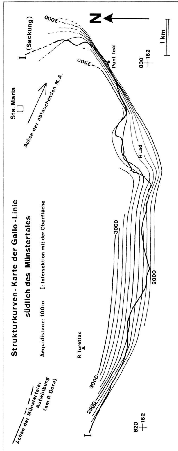
Fig. 17. Strukturkurvenkarte der Gallo-Linie südlich des Münsterals.
