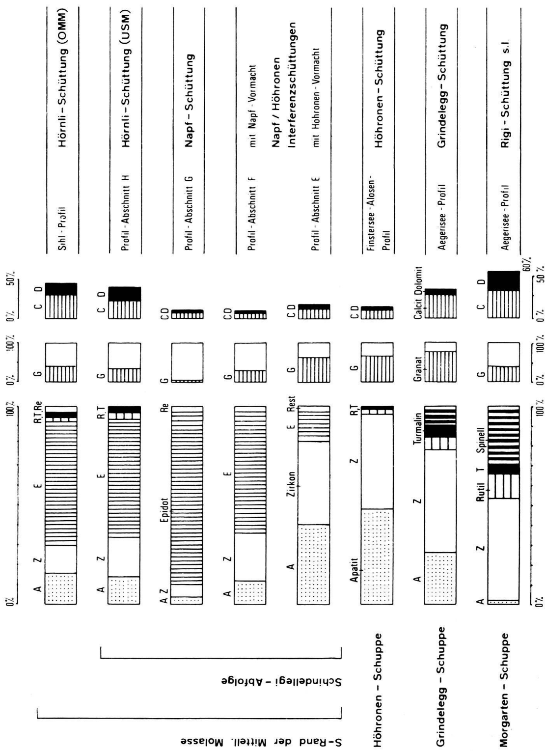
Fig. 22. Sedimentpetrographische Mittelwerte.
