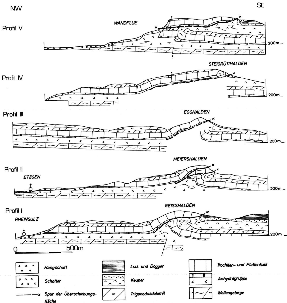
Fig. 2. Tektonische Profile durch die Mettau-Überschiebung zwischen Sulz und Leibstadt (Profilsuren siehe Fig. 1).
