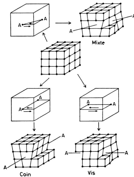
Fig. 12. Représentation schématique d'une dislocation vis, coin et mixte.
