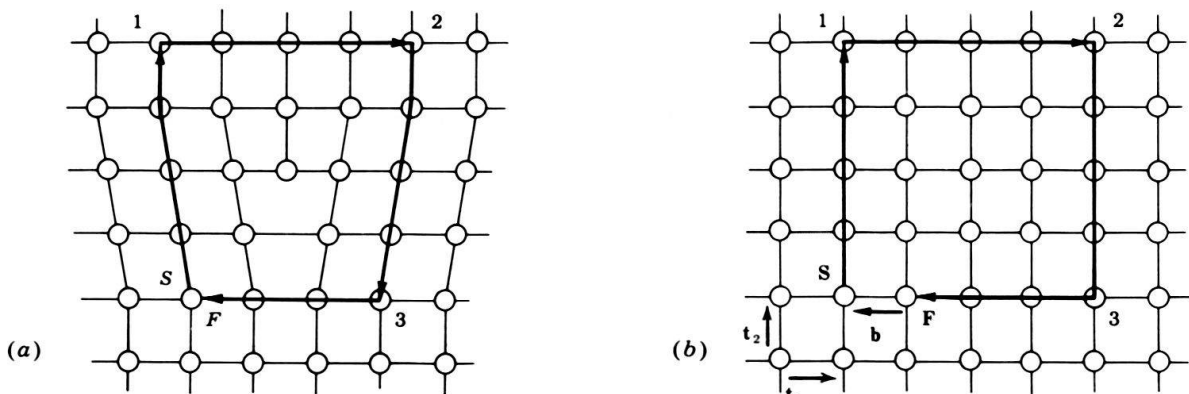
Fig. 17. Définition de vecteur de Burgers.
