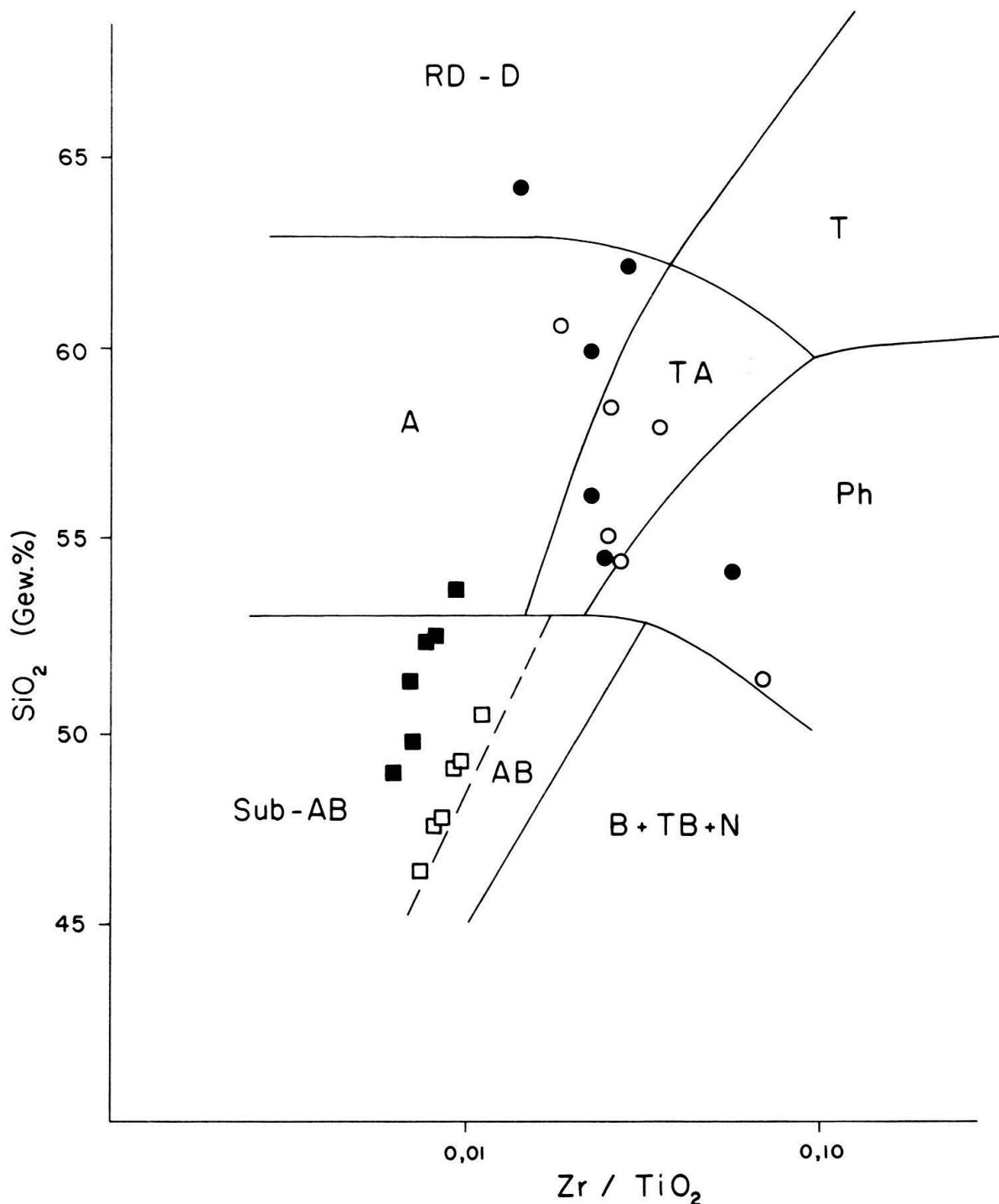
Fig. 6. Korrigierte Analysen der Bentonite im \text{SiO}_2 -Zr/TiO 2 -Diagramm nach WINCHESTER & FLOYD (1977). Symbole: Kreise = vorozeäne Bentonite, Quadrate = eozäne Bentonite, offene Symbole = Korrektur nach STAUDIGEL & HART (1983), schwarze Symbole = Korrektur nach eigenem Probenpaar.
