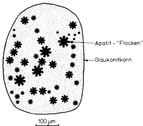
Fig. 7. Aufnahmen mit der Elektronen-Mikrosonde zeigen deutlich, dass die Elementverteilungsmuster von Calcium und Phosphor in einem tektonisch beanspruchten Glaukonitkorn identisch sind. Es dürfte sich somit um «flockige» Apatitverwachsungen handeln, die insbesondere in allen drei Unterkreide-Einheiten G, L und A ausgeprägt vorkommen.
