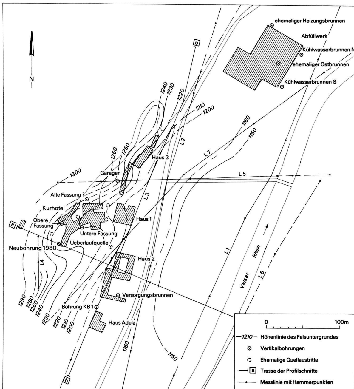
Fig. 3. Plan der Höhenlinien auf der Felsoberfläche im Bereich der Valsener St. Petersquelle, nach Anlage 2 des Berichts Prakla-Seismos GmbH vom 27. April 1981 über refraktionsseismische Messungen in Vals/GR, erstattet an die Valsener St. Petersquelle.
