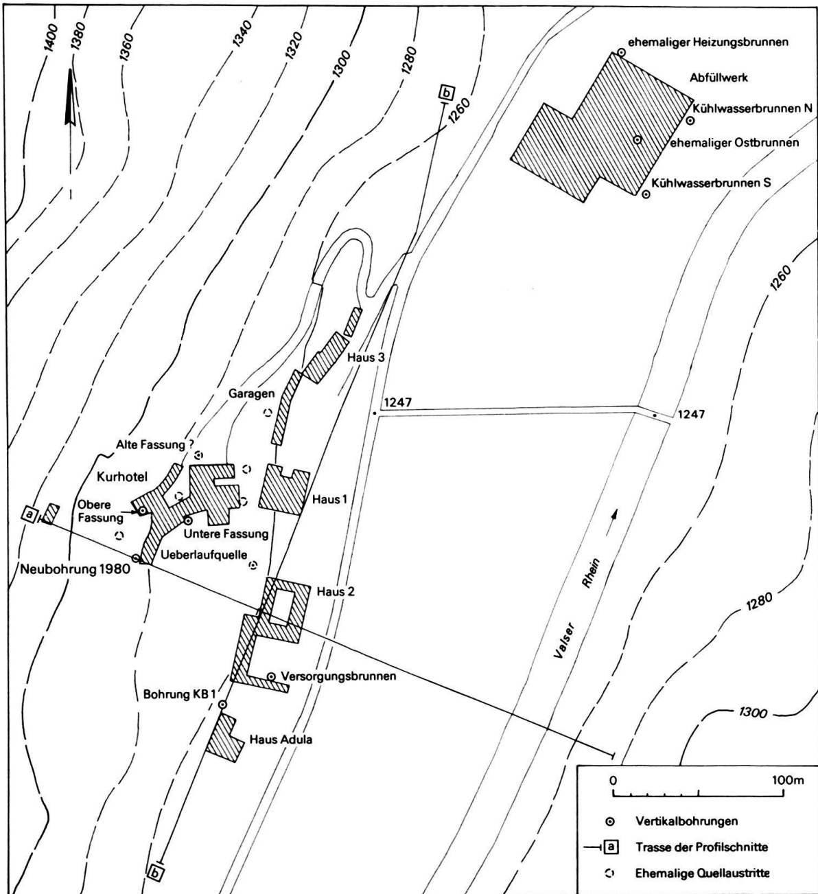
Fig. 2. Situationsplan der Valsen St. Petersquelle und der zugehörigen Gebäude, mit Eintrag der Vertikalbohrungen, der ehemaligen Quellaustritte und den Trassen der Profilschnitte ( a = \text{Fig. 4} , b = \text{Fig. 5} ).
