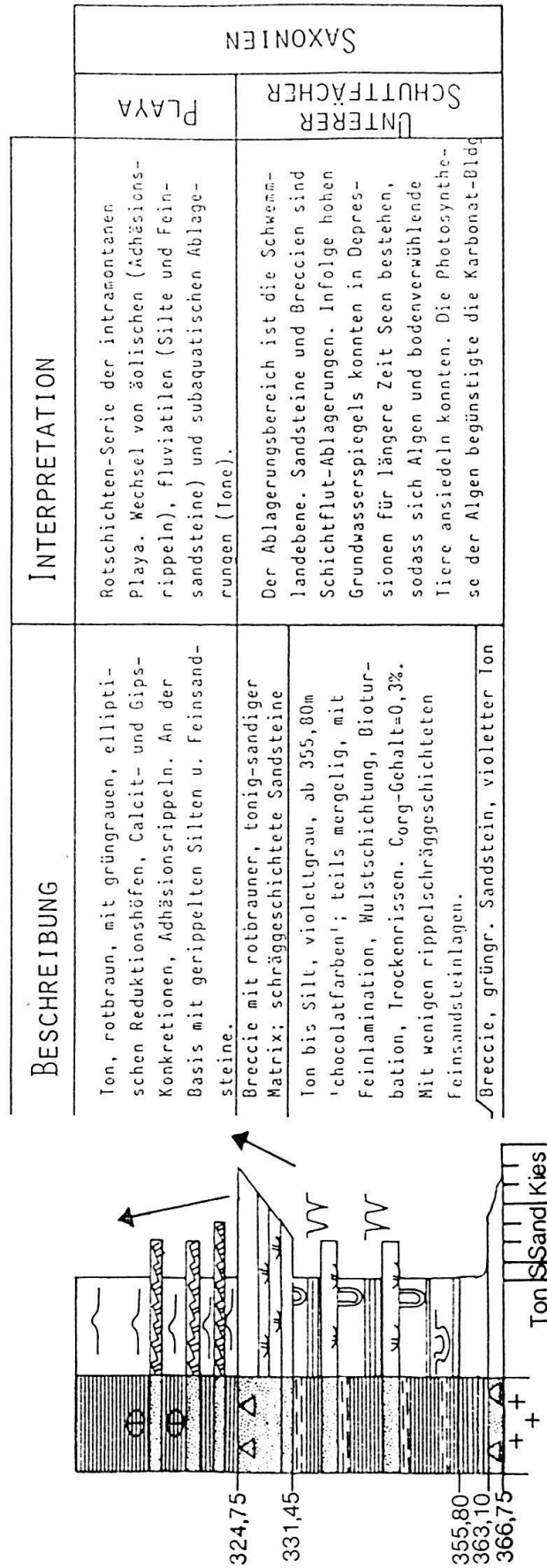
Fig. 9. Sedimentologisches Profil der basalen Sedimente der Bohrung Weiherfeld. Teufenangaben nach MÜLLER (1876, S. 25-26).
