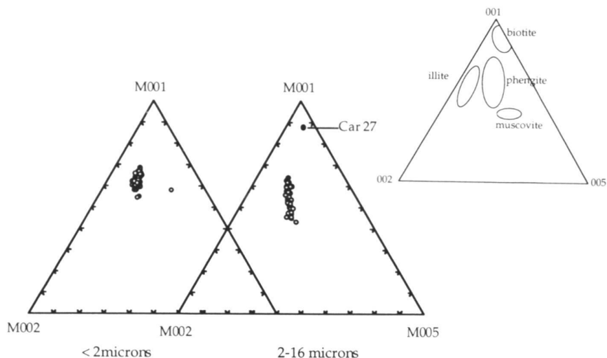
Fig. 5. Représentation graphique des micas selon le diagramme de Rey & Kübler (1983): échantillons Car 27 (en noir) et les échantillons des Bre-guettes (en blanc).
