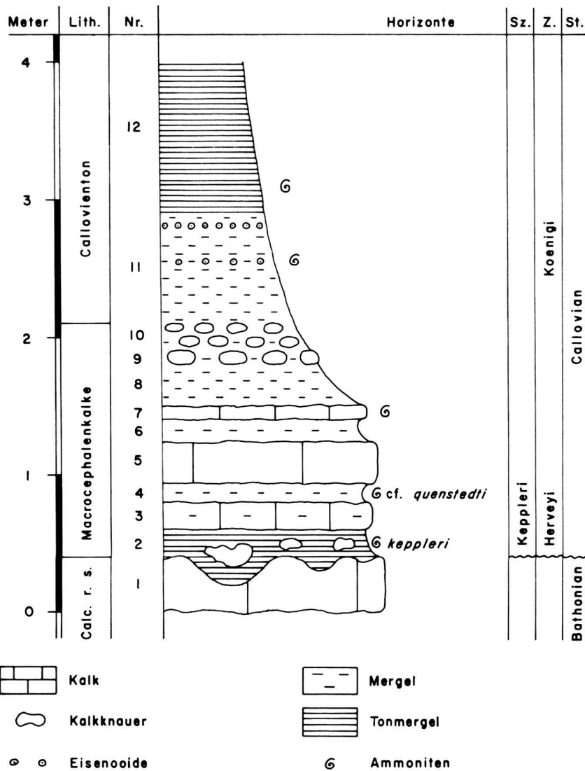
Fig. 1. Profil der Grabung RG 427 in der Tongrube Hinter Chestel bei Liesbergmüli, Liesberg BL. Calc. r. s.: Calcaire roux sableux.
