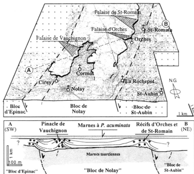
Fig. 2. Situation des falaises de Vauchignon, St-Romain et Orches par rapport aux failles normales délimitant le «bloc de Noly». L'influence synsédimentaire de ces failles est perceptible dans les variations d'épaisseur de la série bajocienne et dans l'implantation des récifs coralliens.
