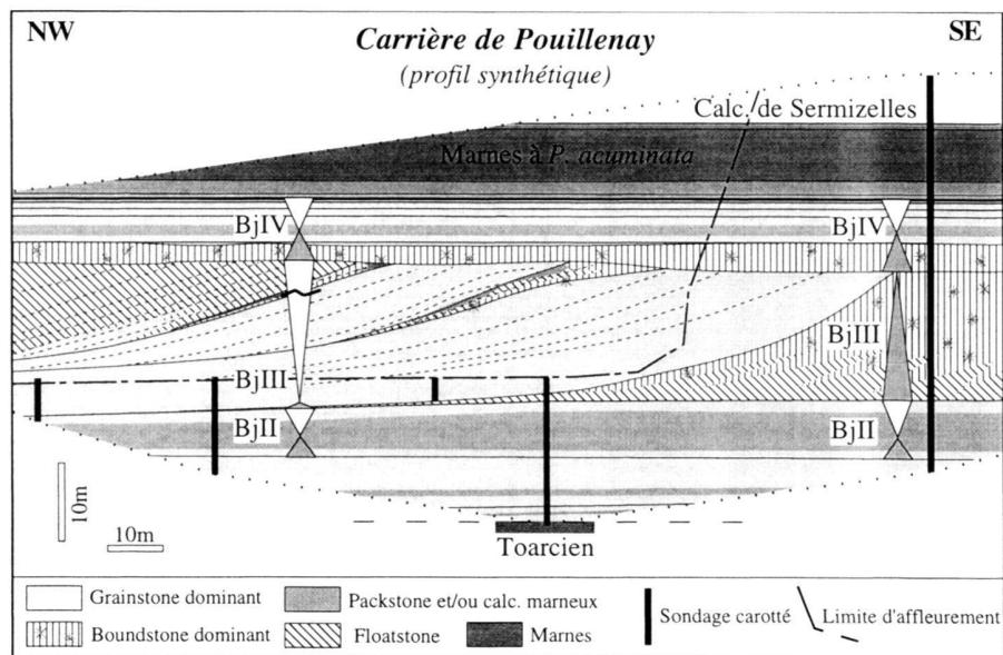
Fig. 6. Distribution des faciès et des discontinuités au niveau de la carrière de Pouillenay. Des sondages carottés complètent les relevés des fronts de taille. Dans la carrière, la séquence BjIII est principalement représentée par des faisceaux progradants mis en place sur le flanc ouest et nord-ouest d'un pinacle corallien reconnu par un sondage carotté effectué au sud-est de l'excavation. Ces faisceaux montrent une alternance de faciès bioconstruits (souvent argileux et uniquement au sommet des talus), de faciès de démantèlement et d'encrinites. Le sommet de ces faisceaux est tronqué par une surface érosive et émergitive qui matérialise le maximum régressif du début de la séquence BjIV.
