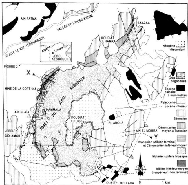
Fig. 1. Localisation schématique (cartouche) et carte géologique simplifiée du J. Kebbouh. Le Quaternaire est en blanc, les fractures en trait fort (supposées en tireté) ; X-Y : localisation de la coupe interprétative synthétique de la Fig. 5.
