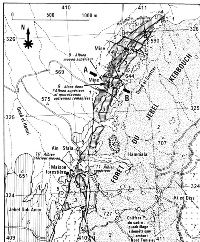
Fig. 2. Carte géologique des versants ouest et nord-ouest du Jebel Kebbouh. Mêmes figurés que pour la Fig. 1.
