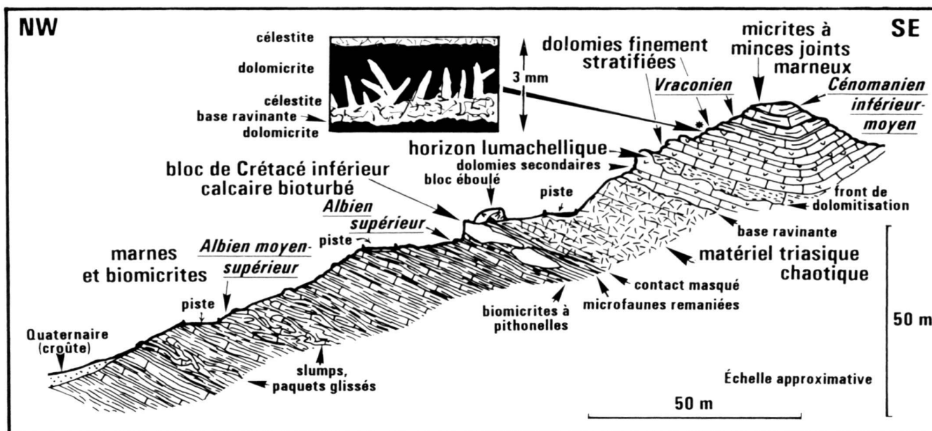
Fig. 3. Coupe géologique synthétique du versant nord-ouest du J. Kebbouch par l'ancienne mine (Kebbouch Asturienne), un peu au sud de la cote 644 (localisée Fig. 2), complétée au-dessus de l'étoile, par une coupe parallèle, passant par la cote 644, 150 m au NW. Cartouche : voir texte.
