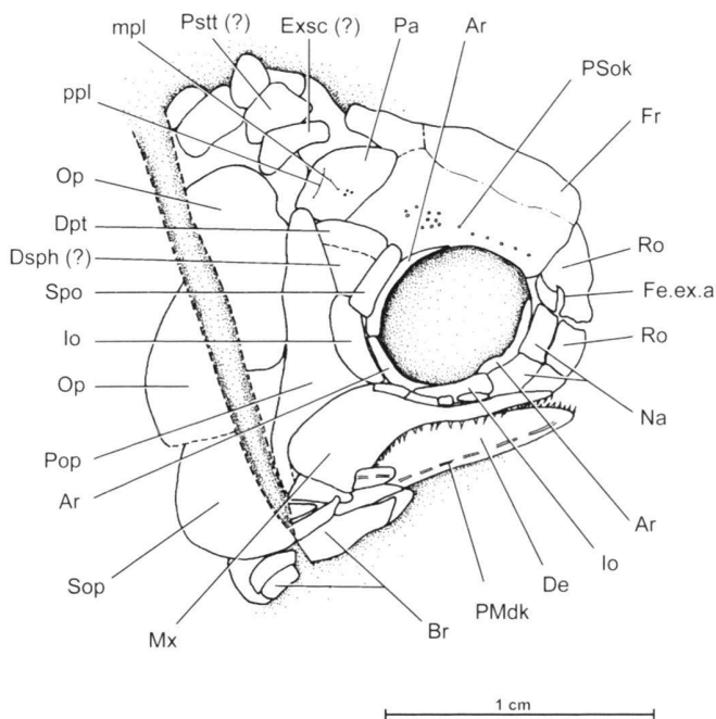
Fig. 19: Peltoperleidus bellipinnis BÜRGIN, 1992. Schädel in Lateralansicht (PIMUZ A/I 2664, Ducanfur- ga 4, Sertig, Davos).
