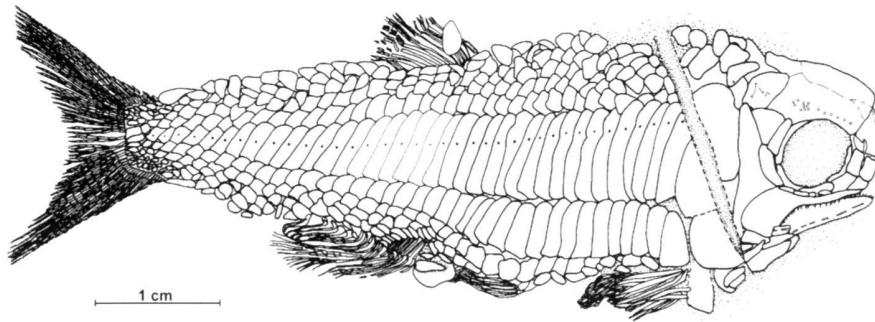
Fig. 18: Peltoperleidus bellipinnis BÜRGIN, 1992. In Lateralansicht (PIMUZ A/I 2664, Ducanfur- ga 4, Sertig, Davos).
