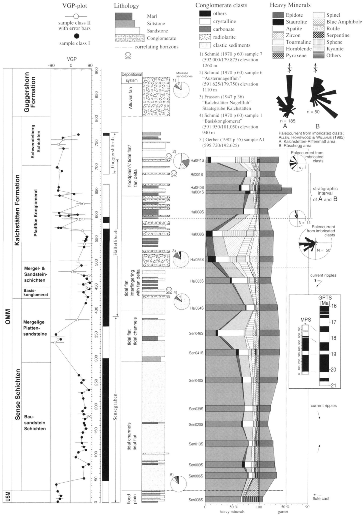
Fig. 6. Lithologic, paleomagnetic- and heavy mineral log of the Sensegraben/Hälttelibach/Guggershörhörnli section.
