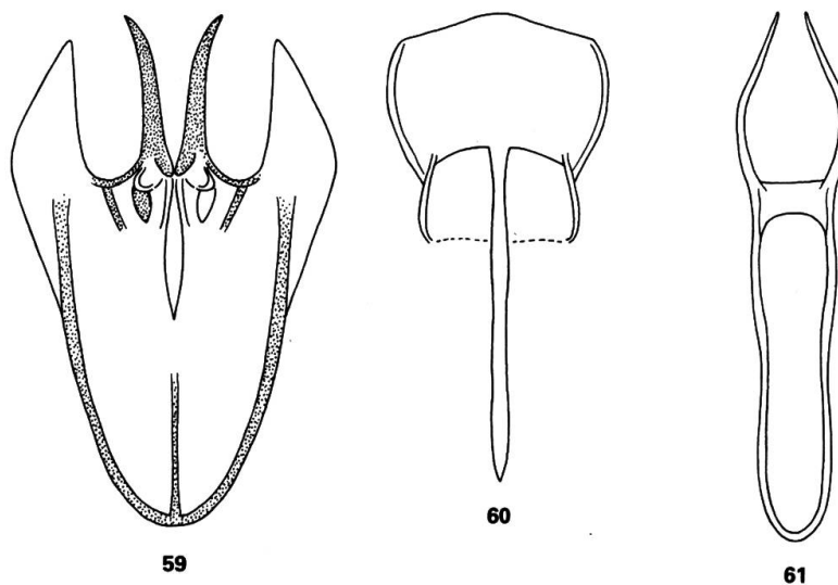
Abb. 59–61: Cyphon unipunctatus n.sp., Holotypus: 59, 9. Sternit. 60, Tegmen. 61, Penis.
