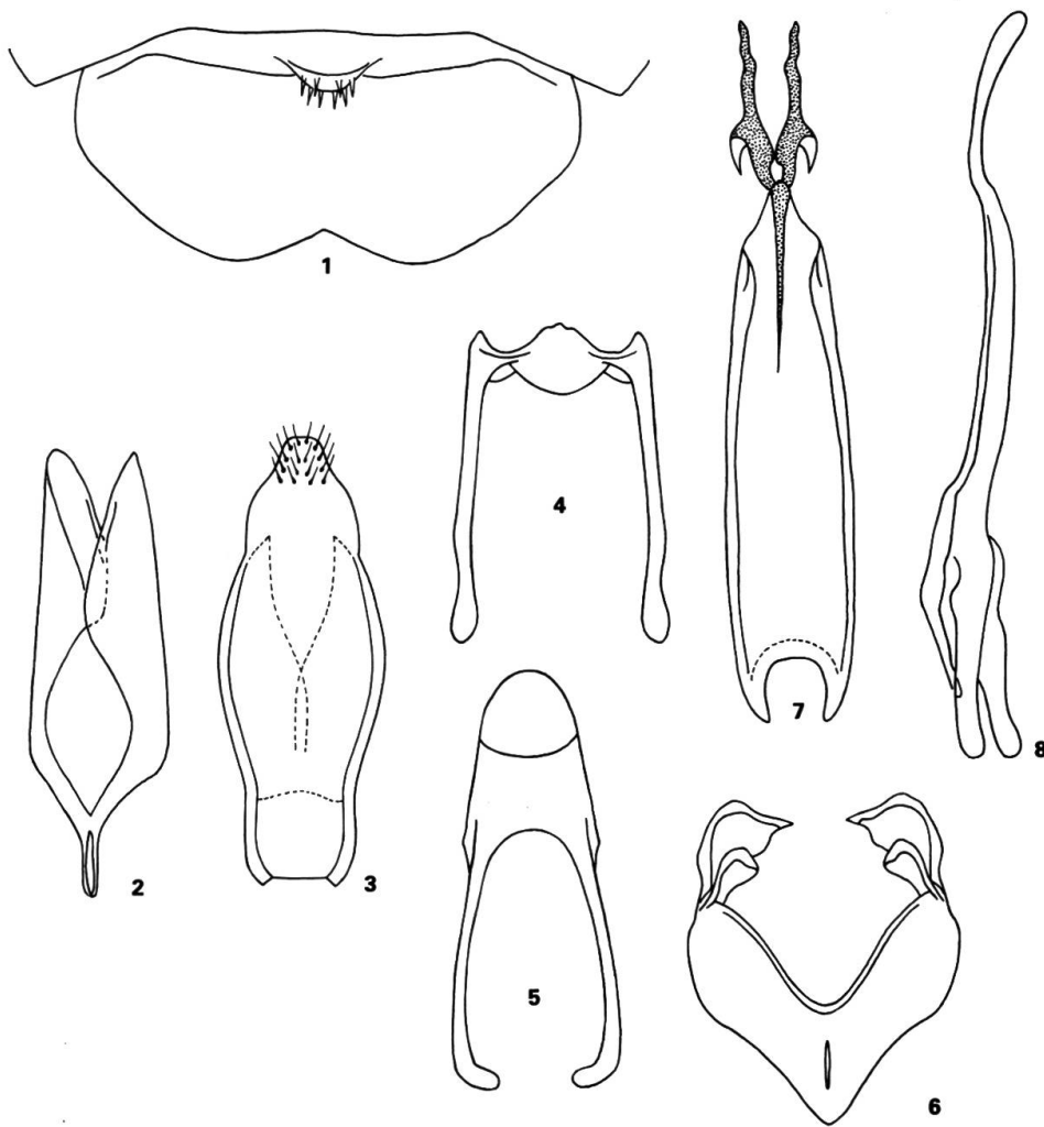
Abb. 1–8: Flavohelodes indubia n. sp., Holotypus: 1, 6./7. Sternit. 2, 8. Sternit, 3, 9. Sternit. 4, 8. Tergit. 5, 9. Tergit. 6, Tegmen. 7, Pars dorsalis penis. 8, Pars ventralis penis.
