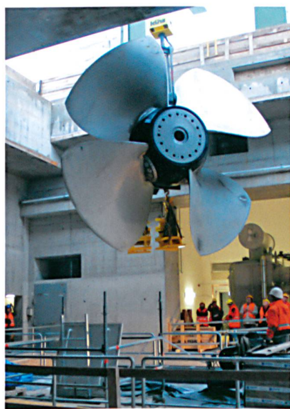
Das Einheben des Laufwerks für die Turbine erforderte millimetergenaues Arbeiten: Es wiegt 60 Tonnen und wurde in einem Stück angeliefert.
