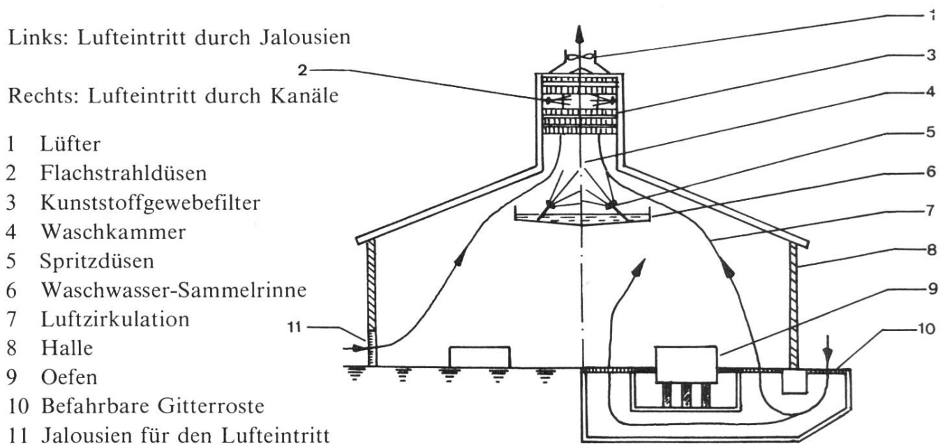
Schema der Hallenablufreinigungsanlage (Nach Moser, 1969)
