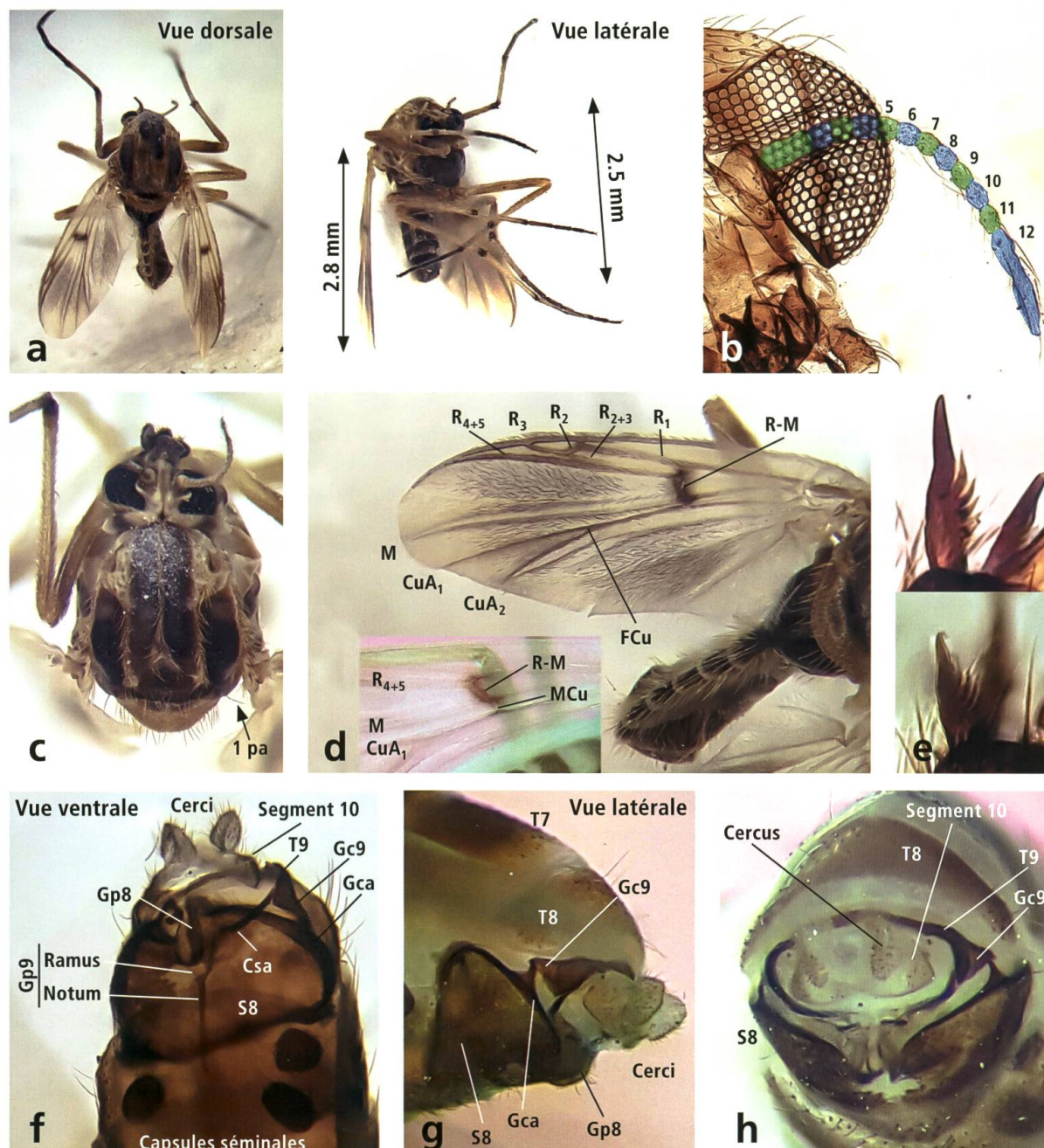
Fig. 1. Femelle de Procladius culiciformis (Lausanne). a ) Habitus. b ) Antenne. c ) Thorax et tête. d ) Aile. e ) Épines tarsales des pattes 2 (image supérieure) et 3 (image inférieure). f ) Terminalia (vue ventrale). g ) Terminalia (vue latérale). h ) Terminalia (vue caudale). Abréviations : Csa = coxosternapodème 9, CuA1 = veine cubitale 1, CuA2 = veine cubitale 2, FCu = racine des veines cubitales, Gc9 = gonocoxite 9, Gca = gonaxopodème, Gp8 = gonapophyse 8, Gp9 = gonapophyse 9, M = veine médiane, MCu = veine MCu, pa = soie pré-alaire, R = veine radiale (de 1 à 4+5), R-M = veine R-M, S8 = sternite 8, T7 = tergite 7, T8 = tergite 8, T9 = tergite 9. (Photos Christian Widmann)
