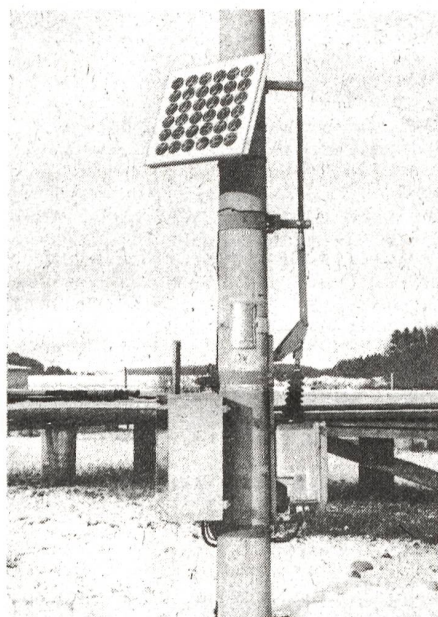
Hier hat das Elektrizitätswerk des Kantons Freiburg Sonnenstrom zur unabhängigen Versorgung eines funktgesteuerten Trennschalters im Mittelspannungsnetz eingesetzt.
