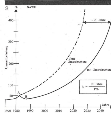
Bild 1: Die Kurven beweisen, dass durch Gewässerschutzmassnahmen der Phosphatgehalt in den Gewässern abgebaut werden konnte. Nun beginnt die Abnahmekurve wieder abzufachen und wird in einzelnen Seen bald wieder ansteigen. Eine tolerable Belastung (gesundes Gewässer) ist aber mit Gewässerschutzmassnahmen nie zu erreichen. Das Übel müsste durch eindeutige Gesetze und konsequente Überwachung an der Quelle erfasst werden.
