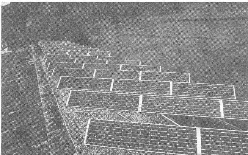
Fotovoltaik und ein 1,8kW-Solargenerator des Ökozentrums Langenbruck produzieren rund 2000 kWh Strom im Jahr - ohne Schadstoffe, ohne Lärm und ohne Strahlung.
