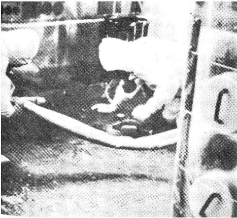
Fig. 10: Schlussdekontamination Dekontamination des PVC-Bodenbelages durch Abhobeln. EIR-Bericht Nr. 559
