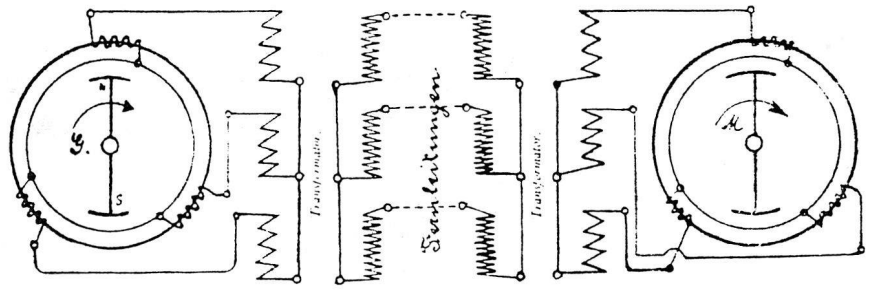
Abb. 12: Haselwander-Schema Drehstromsystem, 1887.
