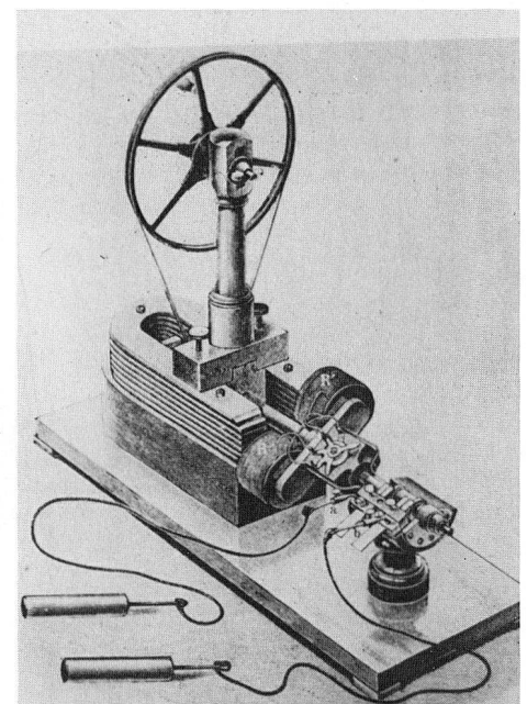
Abb. 2: Störcher's magnet-elektrische Maschine, um 1840.
