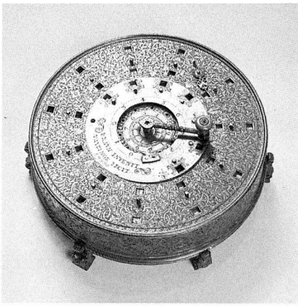
Vier-Spezies-Rechenmaschine von Antonius Braun um 1750 in ornamentiertem Messinggehäuse, im Deutschen Museum. Durchmesser 19,5 cm. Drei Zifferscheiben herausgehoben.
