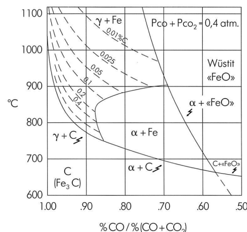
Fig. 1. Das Bauer-Glücksner-Diagramm für Gas - Feststoff - Gleichgewichte im System Fe-C-O-N, bei Gesamtdruck 1 Atm.
