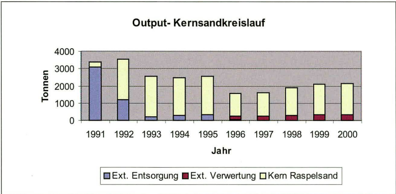
Abb. 8: Output Kernsandkreislauf
