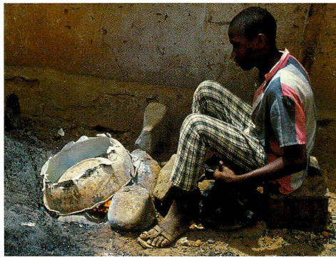
◀ Ofen mit doppeltem Schalengebläse. Die Schalen bestehen aus alten Ölkanistern, die Bälge aus Plastikplanen.
