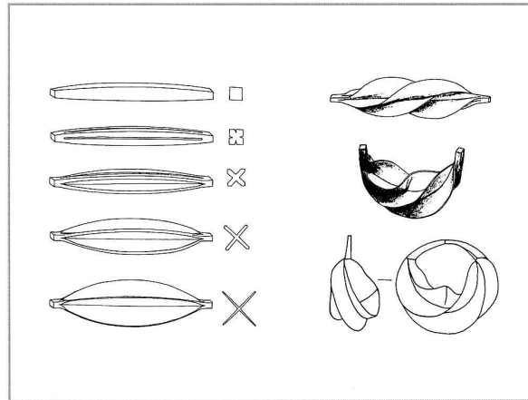
Abb. 34: Schema, Herstellung eines Ohrhings, vom Vierkantstab über den Stab mit kreuzförmigem Querschnitt zum tordierten Endprodukt.
