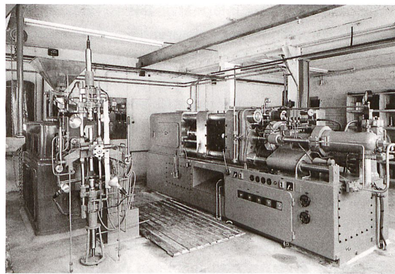
Spritzgussmaschine «Netstal» in der mechanischen Werkstatt für die Kunststoffittings-Entwicklung im Werk II in Schaffhausen, 1955.
