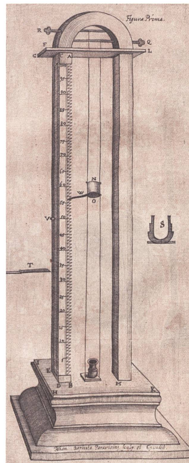
2 Pulverprüfinstrumente, sogenannte épreuves , dienen zur Messung der Qualität von Schwarzpulver.
