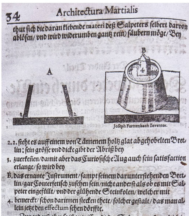
1 Das von Joseph Furtenbach d. Ä. in seinem Traktat «Architectura Martialis» vorgestellte Instrument diente zur Prüfung der Qualität von Salpeter.
