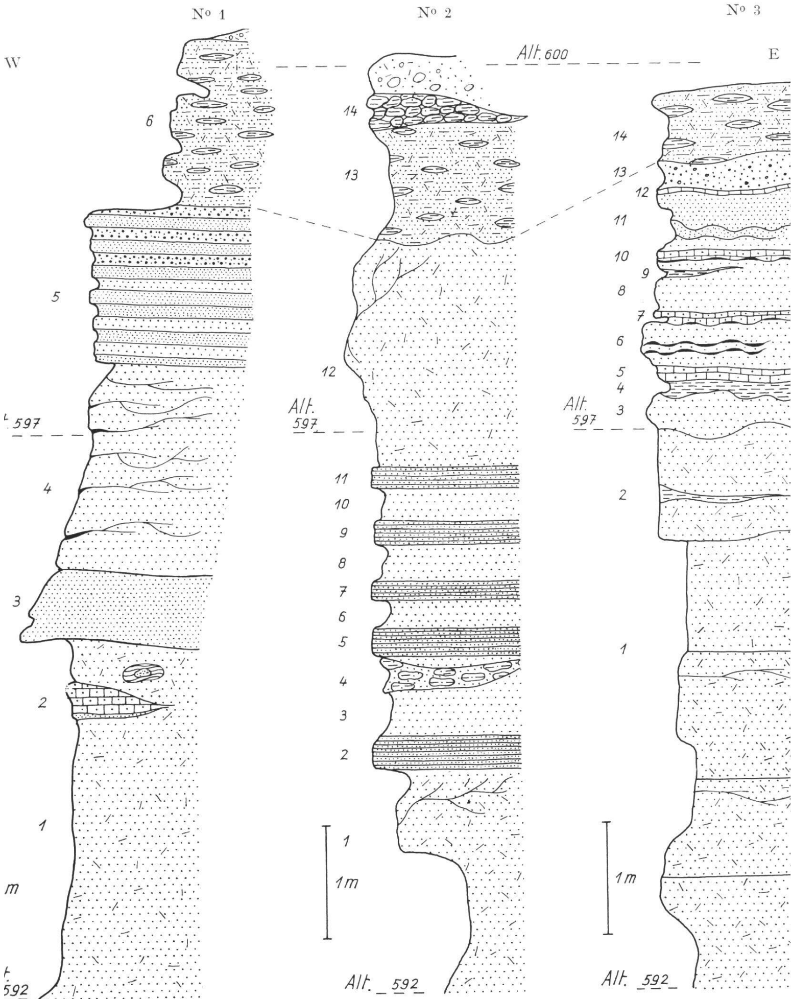
Fig. 15. Coupes s riees de l'affleurement des Roches. Burdigalien inf rieur. Coord. 575,850/192,950.
