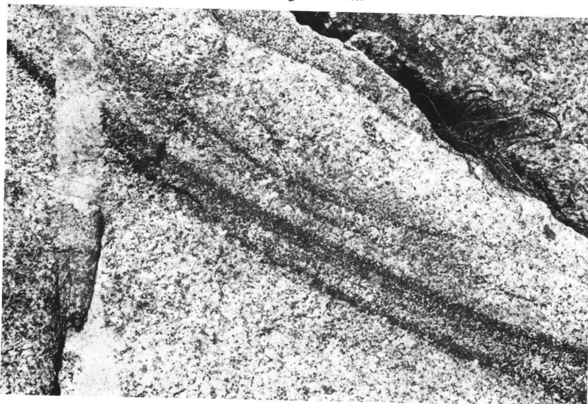
Fig. 17 Granite du Mont-Blanc à grain moyen avec enrichissement de biotite en forme de "Schliere", indiquant une structure primaire dans le granite. Filon aplitique tardif. Alentours de la Cabane d'Orny. Coord. s.: 571590/95205 – 2825 m. Largeur 80 cm.
