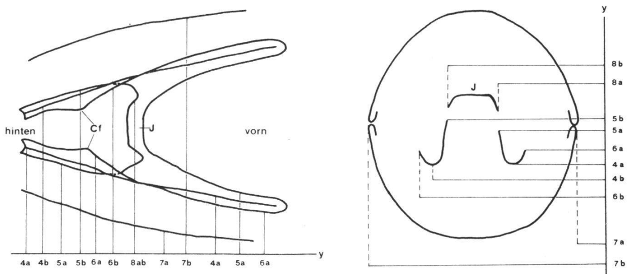
Abb. 2b : Rekonstruktion der Aufsicht. An den Schliffbildern auszumessende Distanzen zwischen den Meßpunkten 4–8 und der y-Achse. a = rechte, b = linke Brachio-podenhälfte. Beschreibung der Meßpunkte siehe Text. Rechts: Beispiel der Ausmessung eines Schliffbildes durch das Jugum (J).
