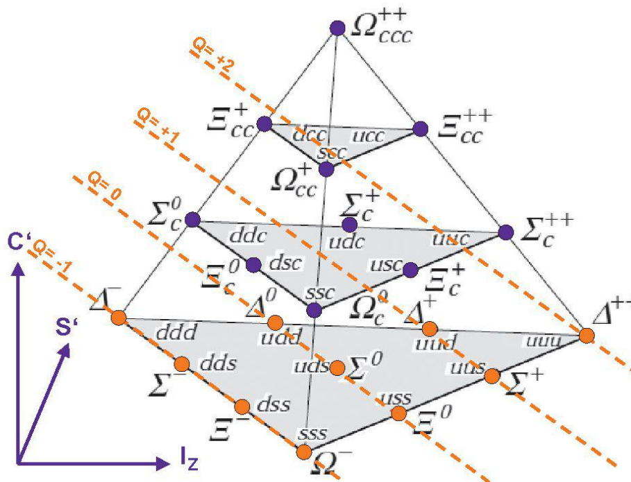
Abb. 8: Übersicht: Klassierung von Elementarteilchen nach Quantenzahlen [PDG]
