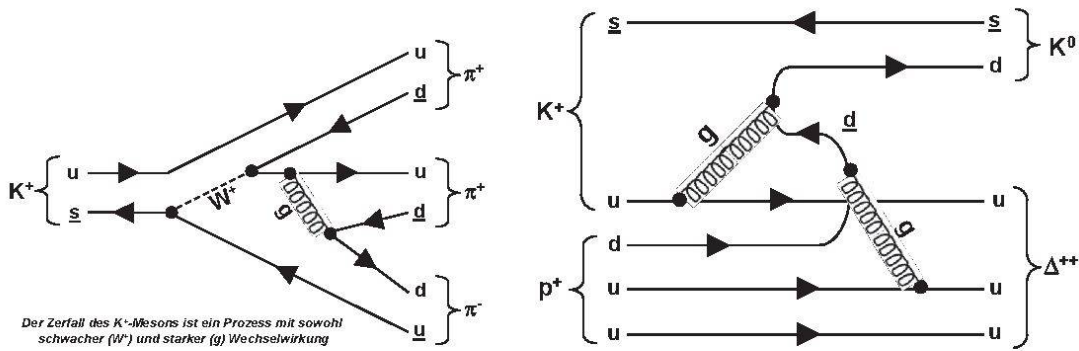
Abb. 17: gemischter Prozesse (K + -Zerfall) und starker Prozess: K^+ + p^+ \Rightarrow K^0 + \Delta^{++}
