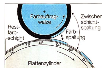
Die Farbübertragung beim wasserlosen Rollenoffsetdruck. Die druckfertige Platte für den wasserlosen Einsatz ist in den nichtdruckenden Partien mit einer Silikonschicht überzogen, die die Farbe abstösst. Die druckenden Teile liegen leicht vertieft und werden aus einer farbaufnehmenden Fotopolymer-Oberfläche gebildet.
