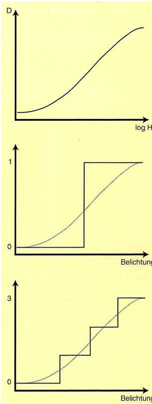
Abb. 4: Von oben nach unten: analoge Aufzeichnung, digitalisierte Aufzeichnung mit 1 Bit und digitalisierte Aufzeichnung mit 2 Bit.
