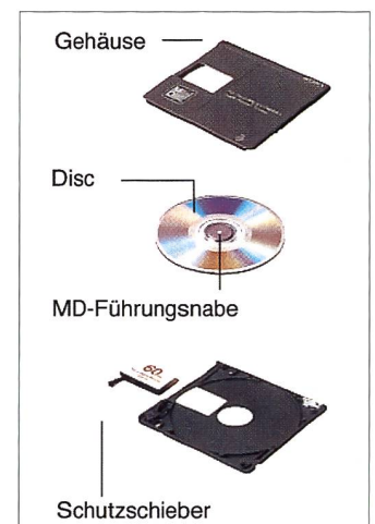
Der Aufbau einer MiniDisc
