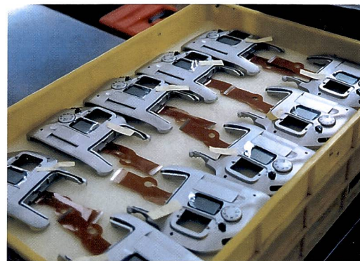
Die fertig montierten Rückwände gelangen lotweise in die Fertigungsstrasse der Pronea S.
