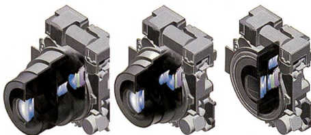
Das neue Pentax Sliding Lens Systems: Die Animation zeigt, wie sich die mittlere Linsengruppe beim Einziehen des Objektivs nach oben verschiebt.
