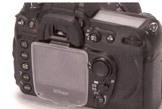
Bascule multifonctions confortable à droite de l'écran pour la mise au point de l'autofocus.
