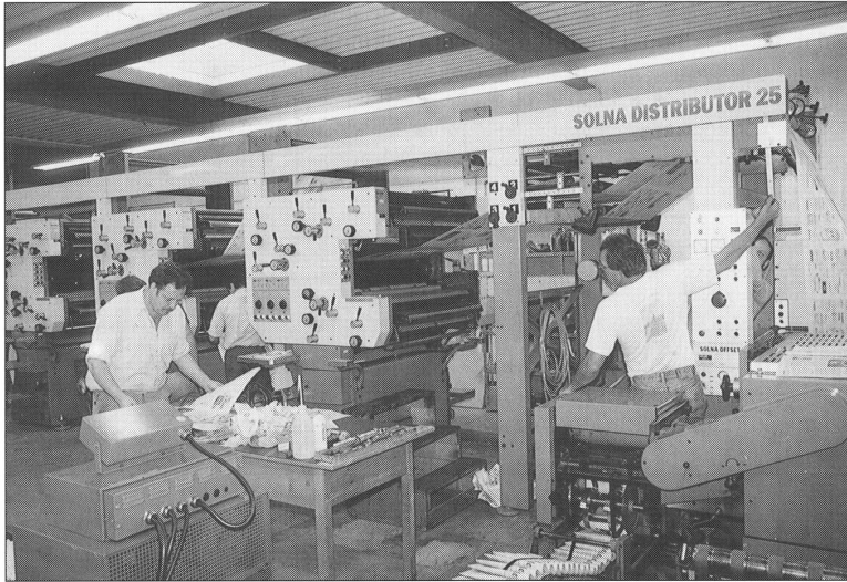
Neue Zeitungsrotations- Offsetmaschine SOLNA D-25, auf welcher 24 Seiten zweifarbig oder 16 Seiten vierfarbig gedruckt werden können.
