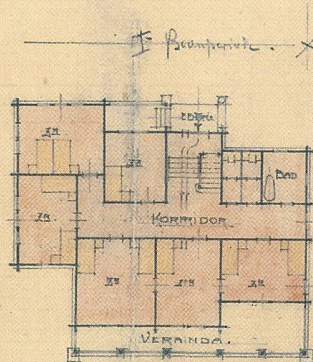
PARTERREGRUNDRISS.
