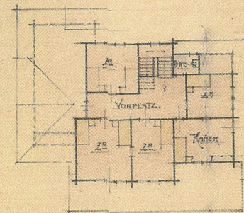
DACHSTOCKGRUNDRISS.
