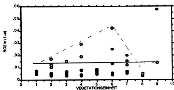
Fig. 4.4. Nitrit
