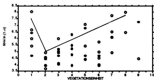
Fig. 4.5. Ammonium
