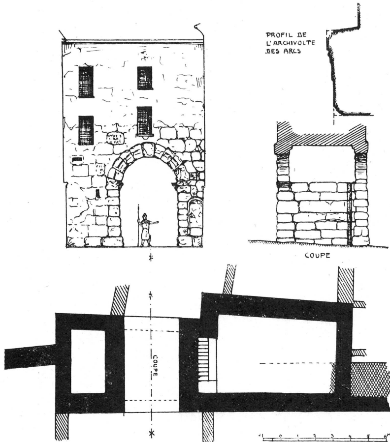
Porte romaine du Bourg-de-Four, d'après M. L. Blondel.
