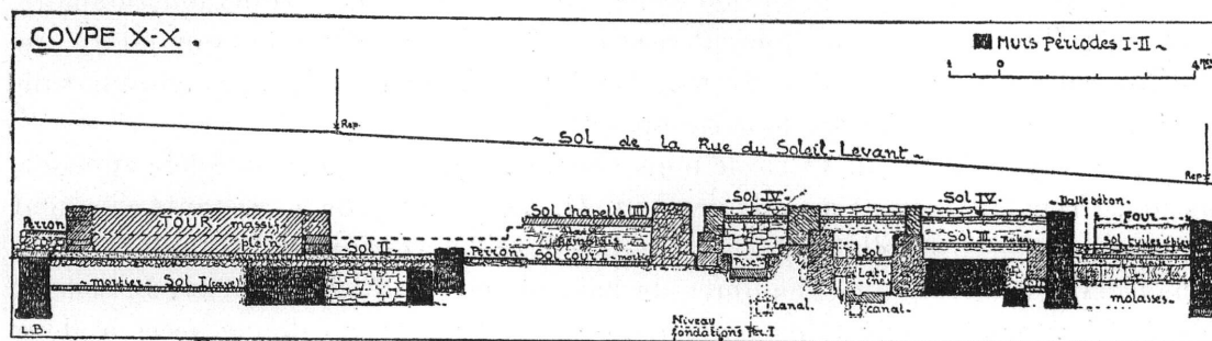
FIG. 2. — Coupe suivant la ligne X-X des fondations sous la rue du Soleil-Levant.
