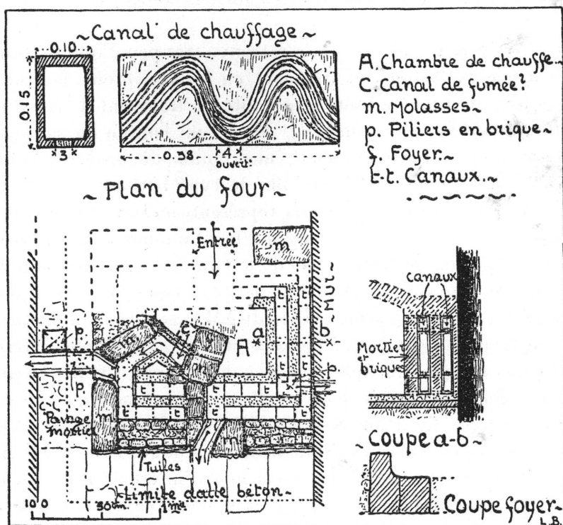
FIG. 8. — Plan, coupe et détails du four.
