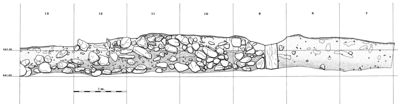
△ ◁ Figure 9. Stratigraphie n° 10.
