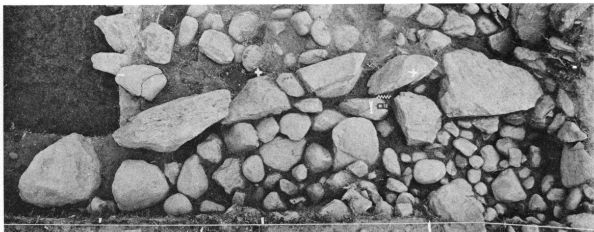
Figure 19. Apparition de la couche 2B2 dans le quadrant 1.
