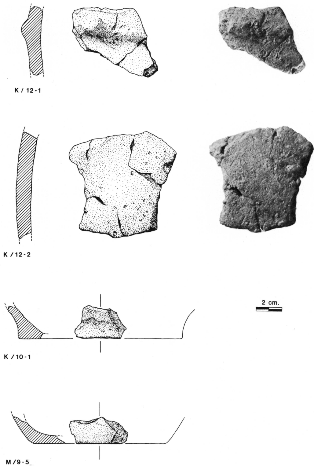
Figure 26. Céramique épaisse avec cordon, fragments de fonds.
