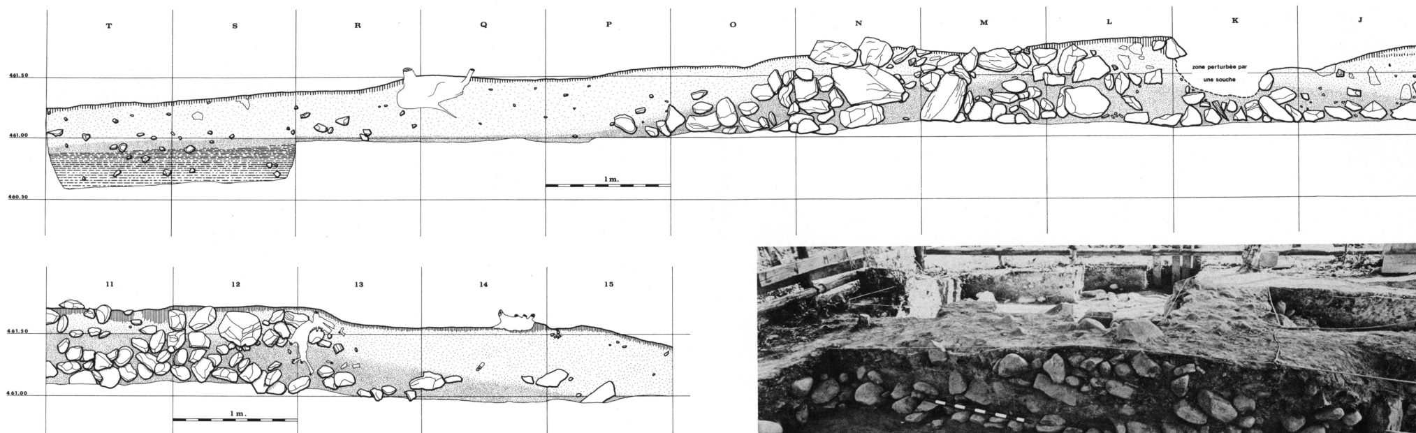
Figure 8. Stratigraphies n° 1 (en haut) et n° 2 (en bas).
