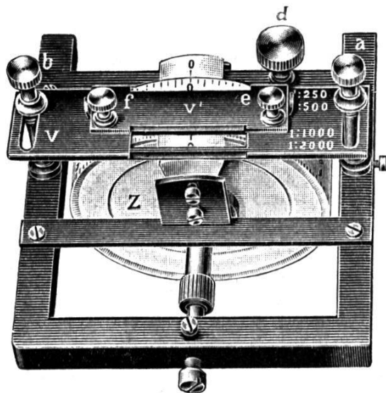
mit Schieber-Verdeckung
