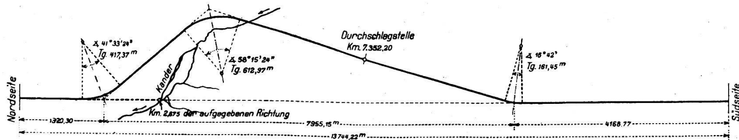
Fig. 2. Längenprofil und Situation des Lötschbergtunnels. Länge 1 : 100,000. Höhen 1 : 5000.
