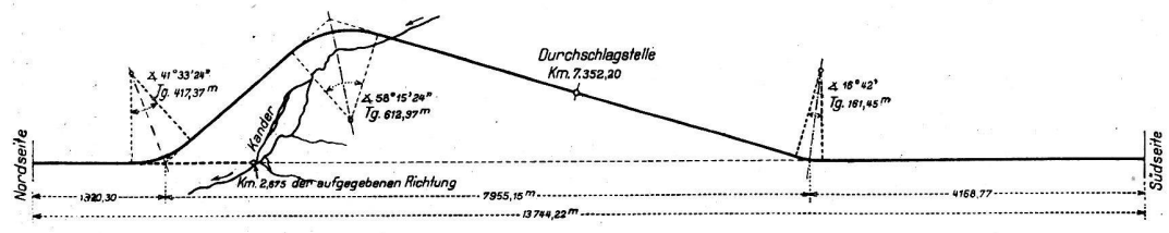
Fig. 2. Profil en long et situation du tunnel du Lötschberg. Longueur 1:100,000. Hauteurs 1:5000.
